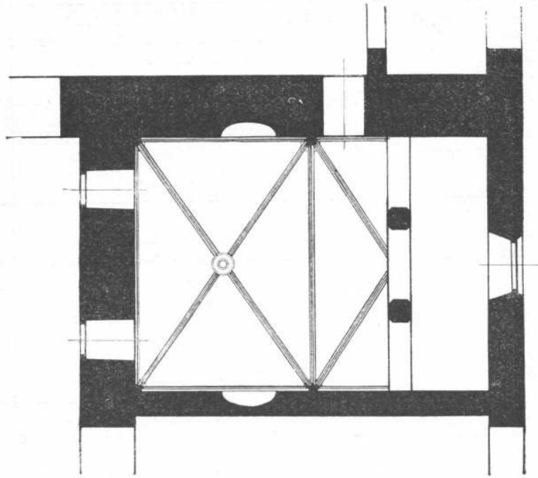
Tlocrt kapele.
