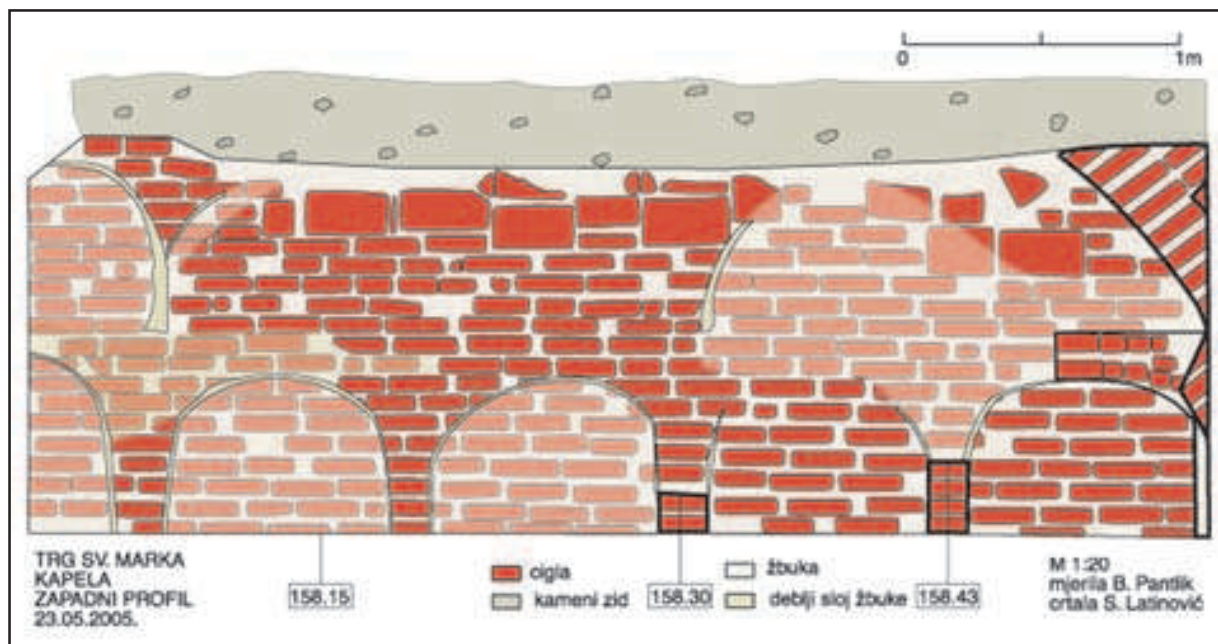
Trg sv. Marka, kapela sv. Fabijana i Sebastijana, kriptna, pogled – zapad (crtež: S. Latinović)
